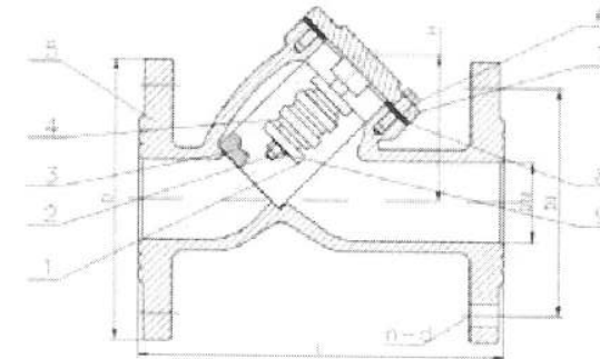
Габаритные размеры, конструкция фильтра ФМФч
