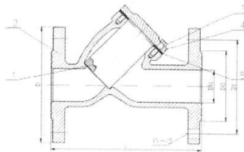
Габаритные размеры, конструкция фильтра ФСФч
